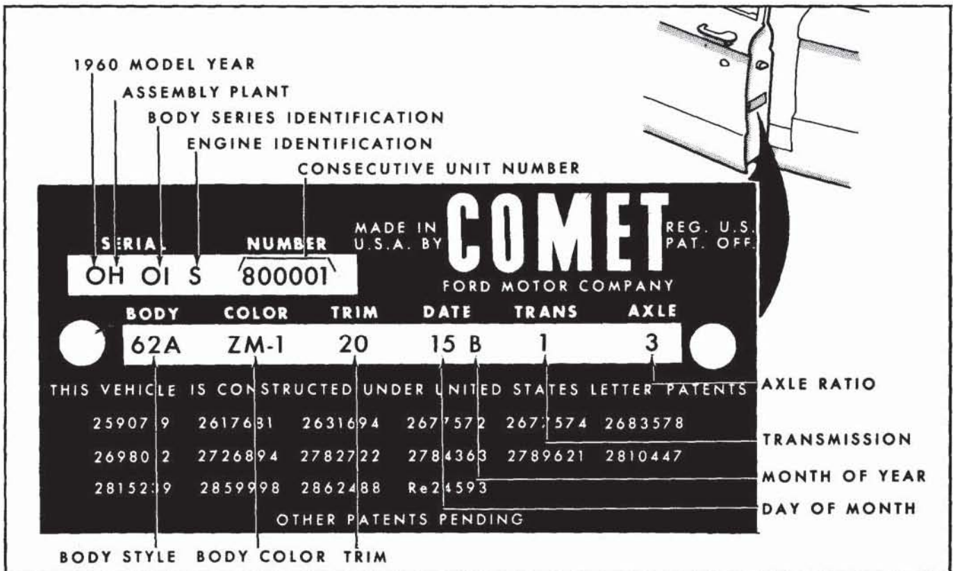
FIG. 7—Patent Plate—(60C-8048)
